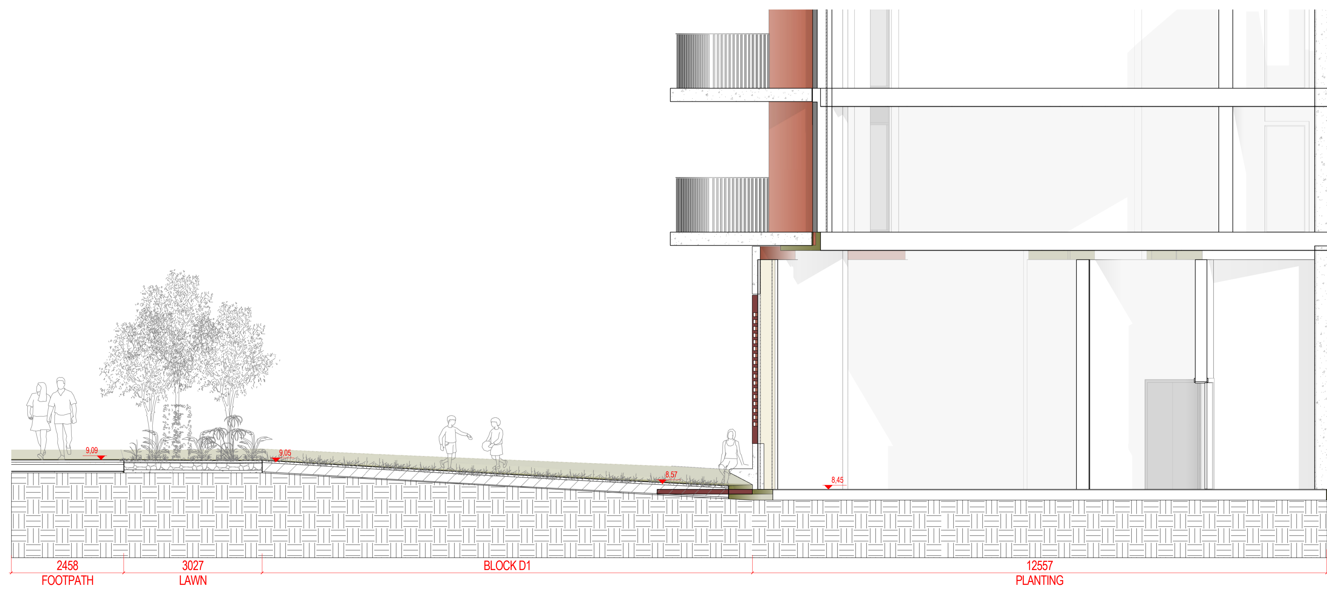
2 SECTION 75 1:50 @A1
